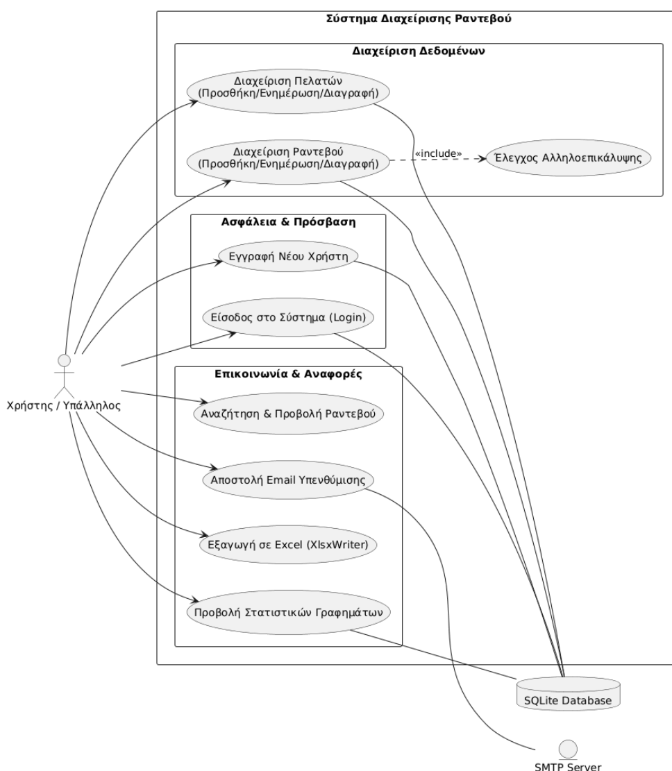
Εικόνα 1: Διάγραμμα αρχικής σχεδίασης use case
