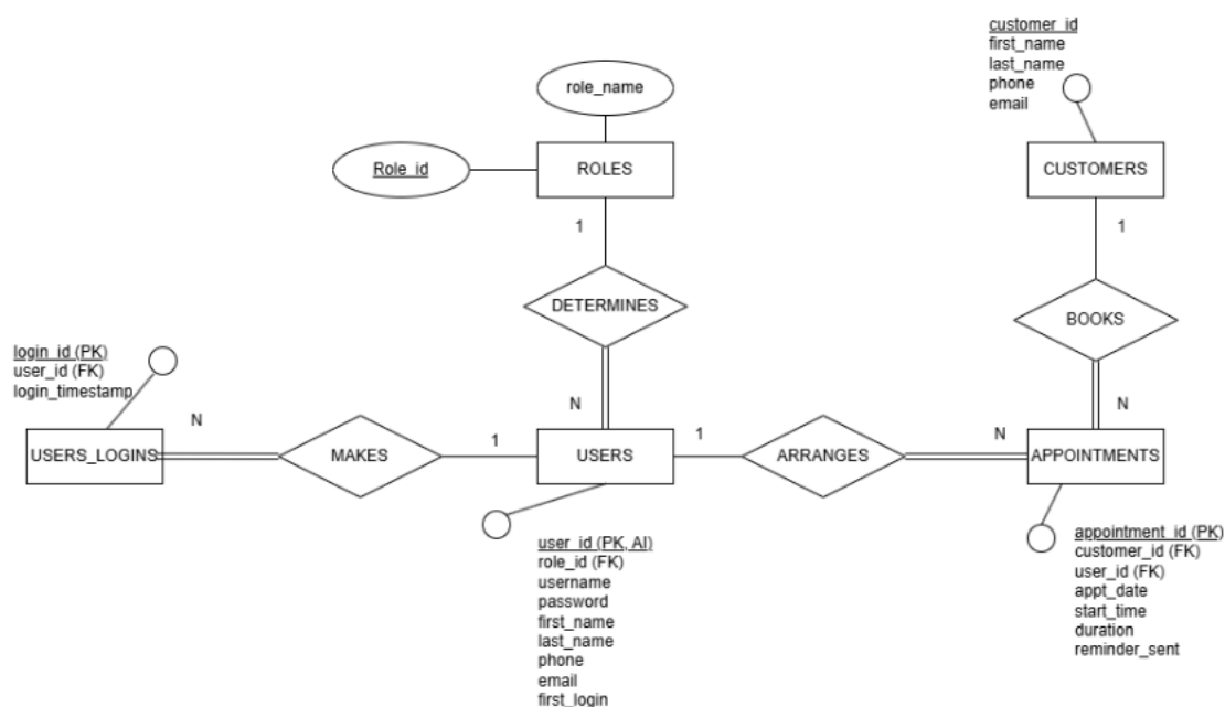
Διάγραμμα 1: Διάγραμμα οντοτήτων-συσχετίσεων αρχικής σχεδίασης
